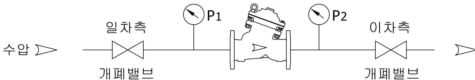
그림 5 내압 시험 장치의 보기
