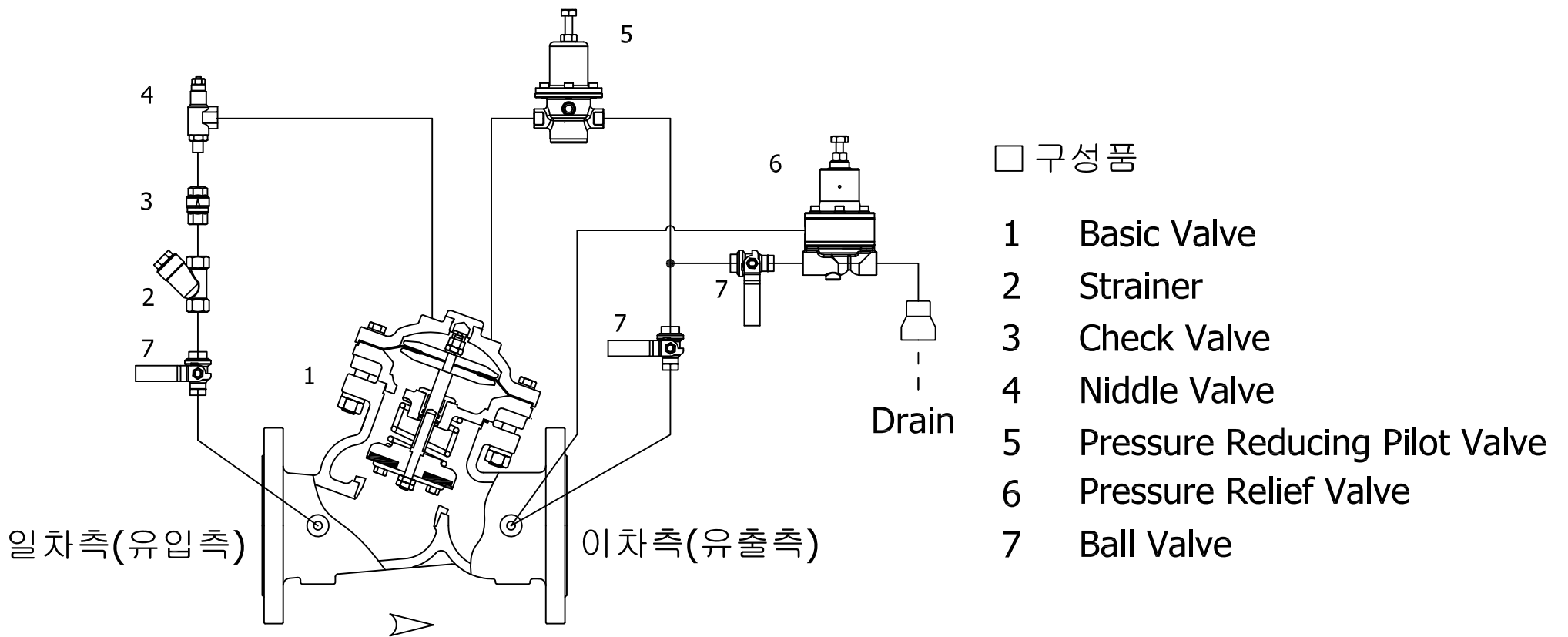
그림 4 감압밸브의 제어 배관도
