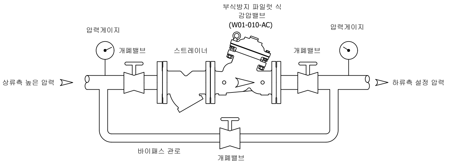
그림 2 부식방지 파일럿 식 감압밸브(W01-010-AC)의 표준 배관도
