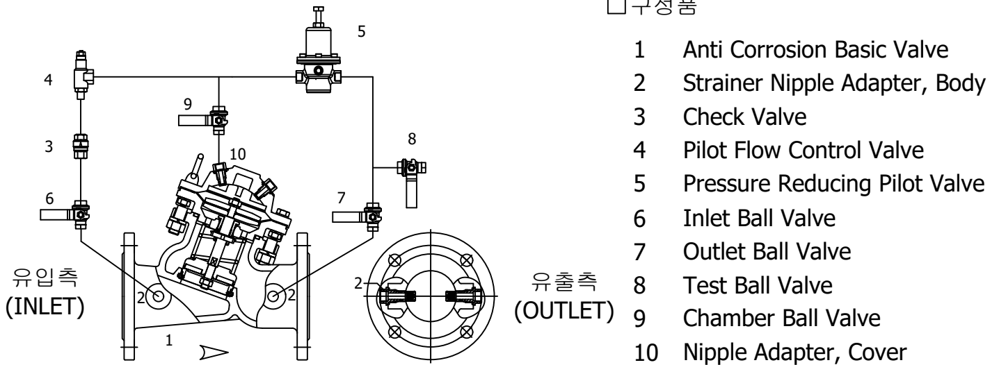
그림1 부식방지 파일럿 식 감압 밸브(W01-010-AC)의 제어 배관도
