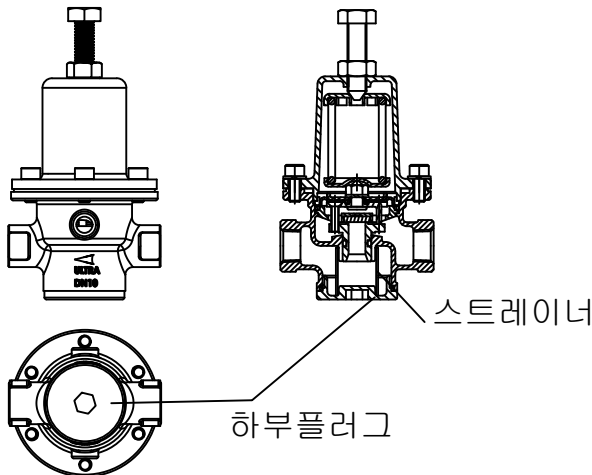
그림 4 파일럿 감압밸브(5)의 형상 및 분해 부품
