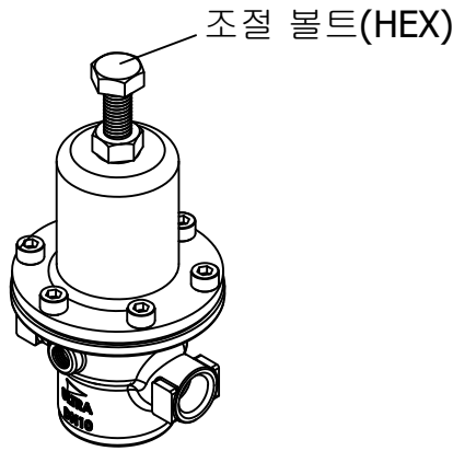
그림 3 파일럿 감압밸브(5)의 압력 조정 방법
